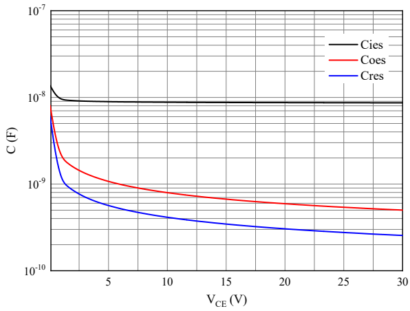
图 9. 电容特性
