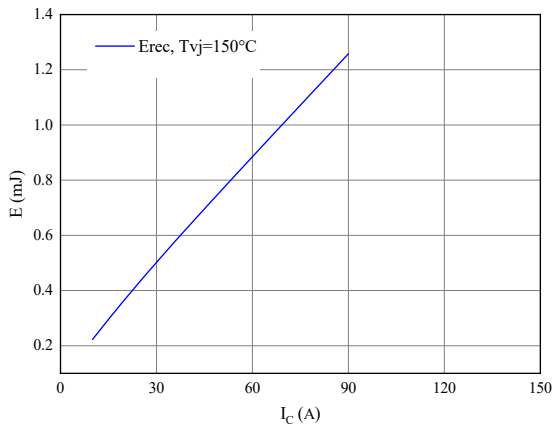
图 7. 开关损耗 二极管 Figure 7. Switching losses of Diode R_{Gon}=1.8\Omega, V_{CE}=400V
