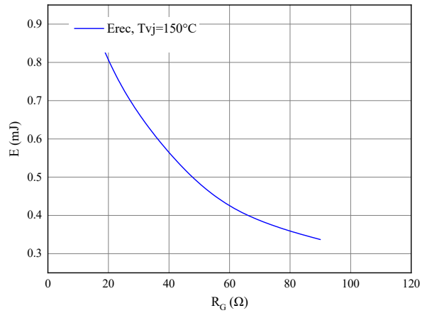
图 8. 开关损耗 二极管 Figure 8. Switching losses of Diode I_F=60A, V_{CE}=400V
