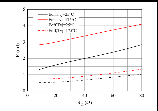
图 8. 开关损耗
