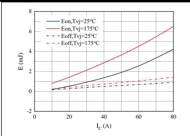
图 7. 开关损耗
