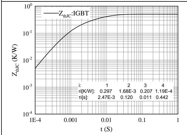
图 11. 瞬态热阻抗 IGBT
