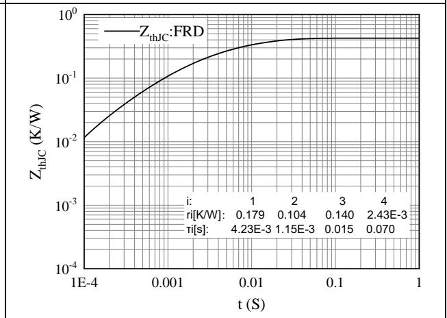
图 12. 瞬态热阻抗 FRD
