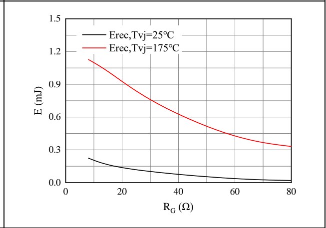
图 10. 开关损耗 二极管
