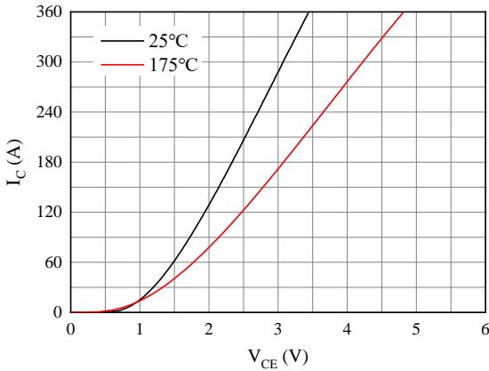
图 3. 典型输出特性 ( V_{GS}=15\text{V} )
