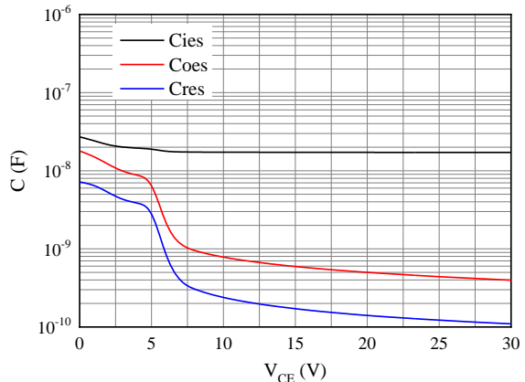
图 6. 电容特性
