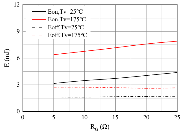
图 8. 开关损耗
