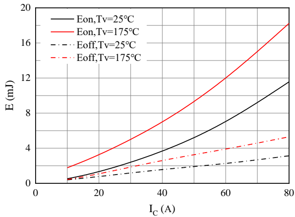
图 7. 开关损耗
